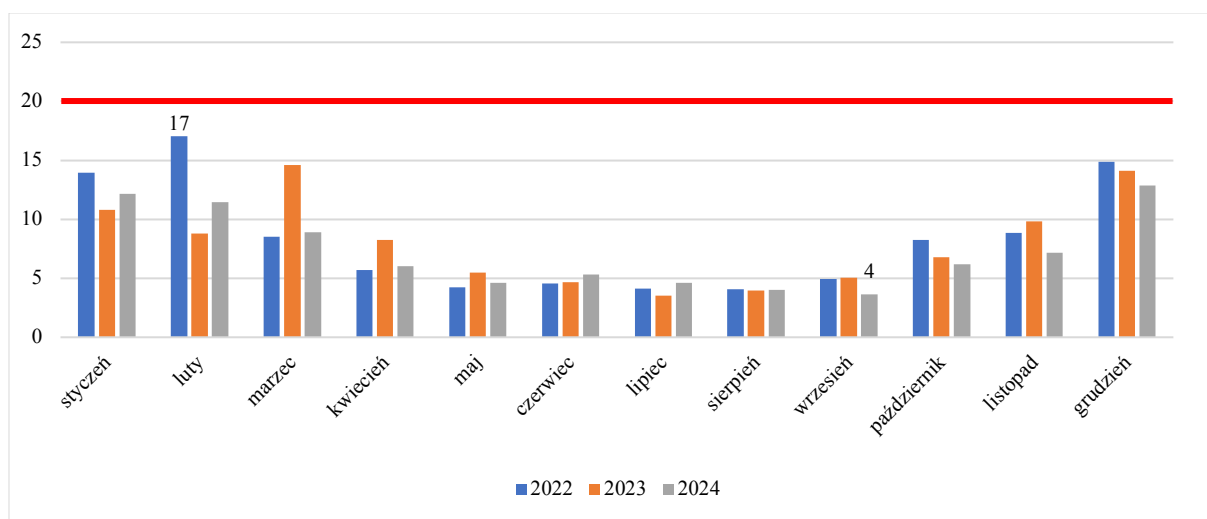
Rysunek 2 Średnie stężenie dwutlenku siarki na stacji w Ustroniu w latach 2022–2024 (µg/m 3 )
